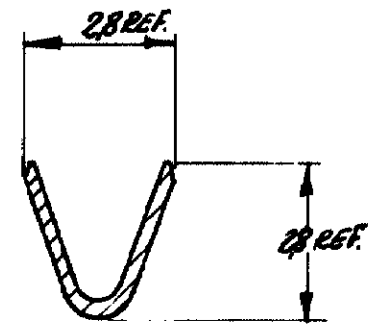
SECCÃO A-A ESC. 8:1
