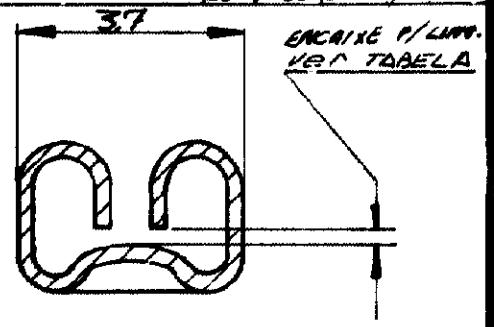
SECCÃO B-B ESC. 8:1
